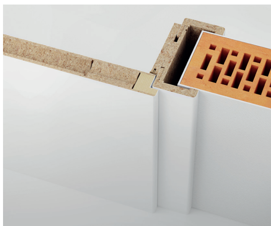
Dveře falcové, hrana dveří oblá, zárubeň oblá / oblá
